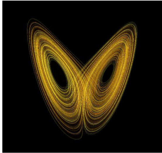
Ο ελκυστής του Λόρεντζ (διάγραμμα πεταλούδας)
